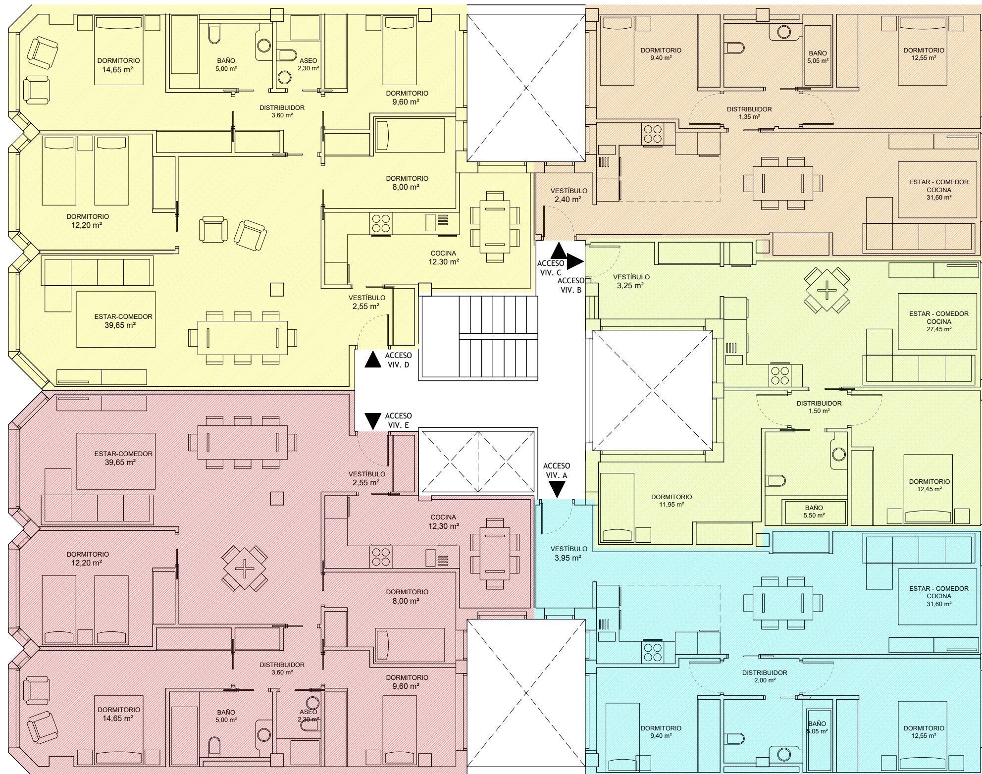
PLANTA TIPO
